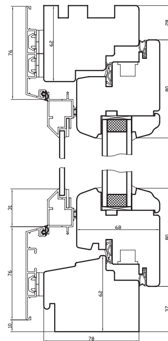
2+1 FÖNSTER RITNING
