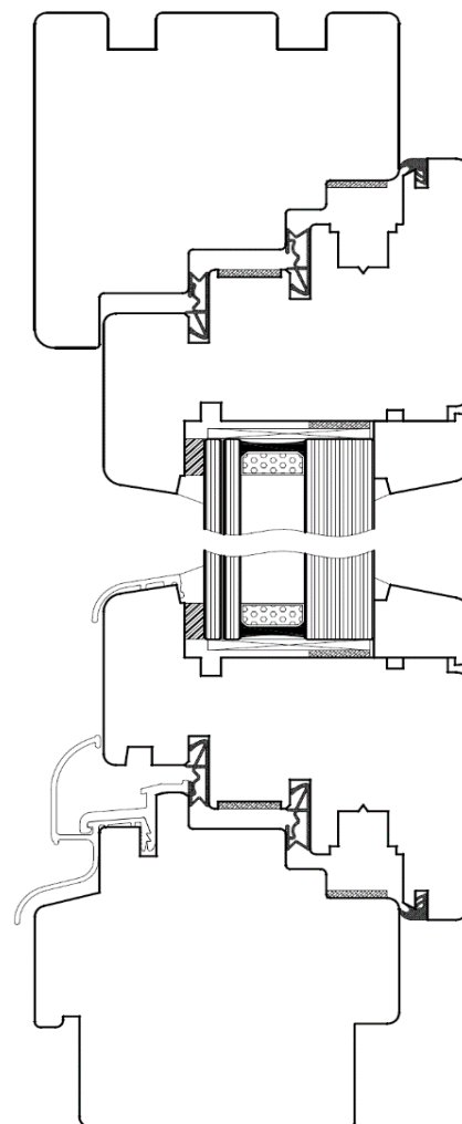
EC/90 EI30 TRÅ RITNING
